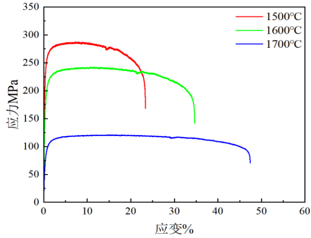
图 6 钨铌合金拉伸应力-应变曲线
