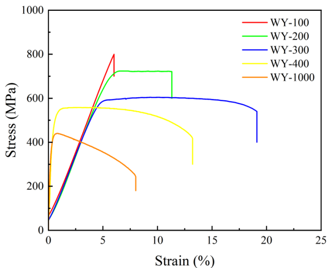
图 8 钨钇合金拉伸应力-应变曲线
