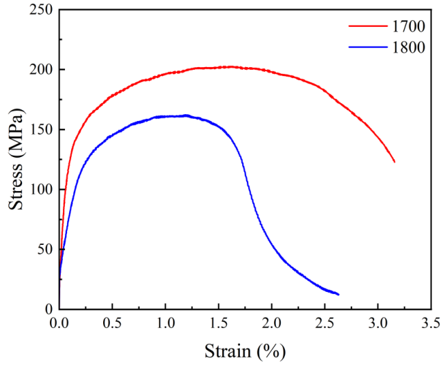
图 5 纯铌拉伸应力-应变曲线
