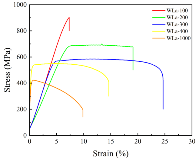
图 7 钨铜合金拉伸应力-应变曲线
