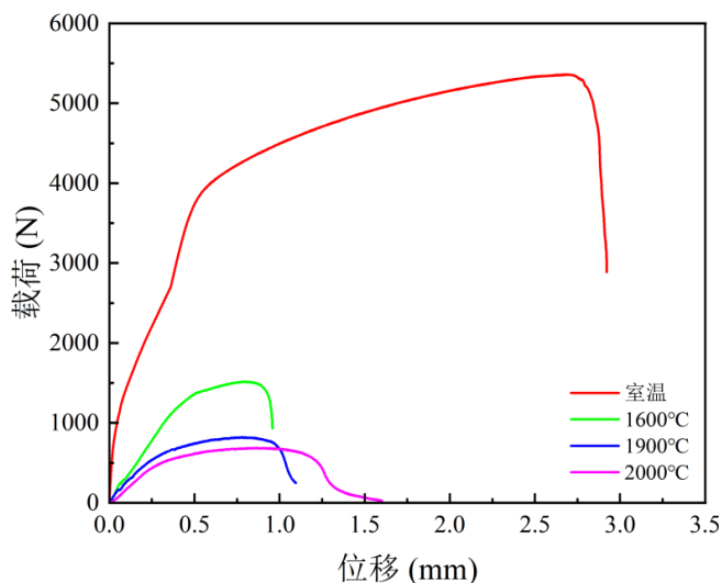
图 9 纯铪拉伸载荷-位移曲线
