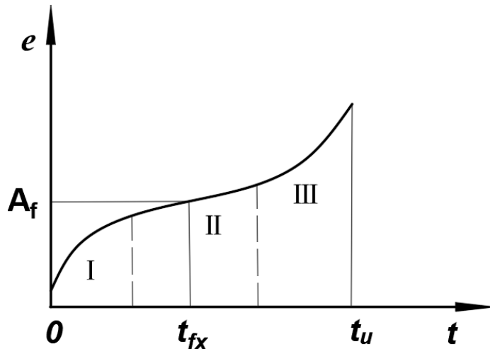
图 4 典型蠕变应变-时间曲线图
